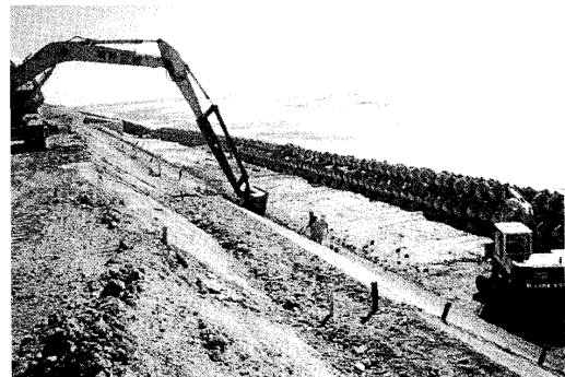
写真 1-3 のり面整形
