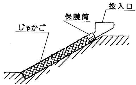
図 1-5 重機による中詰め方法
